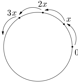
Рис. 12. К теореме Вейля.
